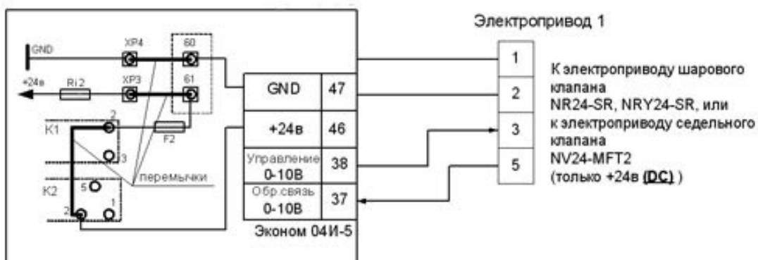
Рис. 9.12 – Схема подключения электропривода «Belimo» с аналоговым управлением 0-10В 1-го канала
