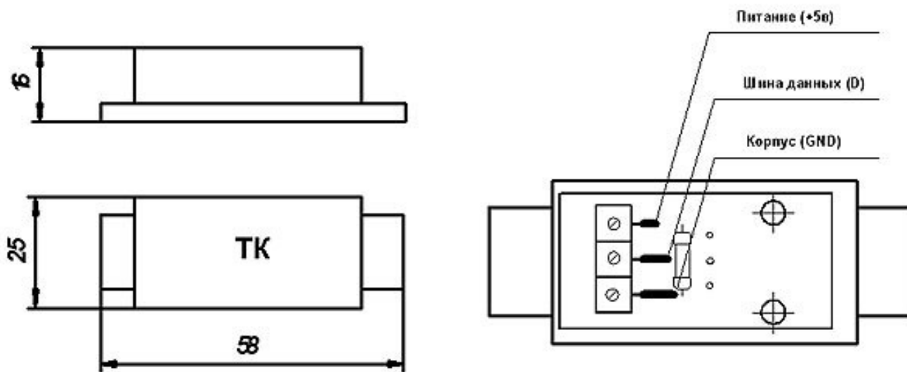
Рис. 6.19 – Общий вид и габаритные размеры термодатчика контактного
