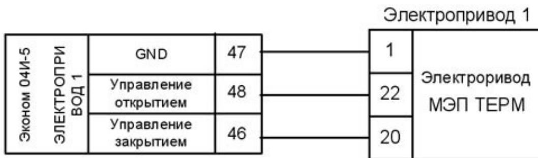
Рис. 9.10 – Схема подключения электропривода 220В МЭП ТЕРМ с трехточечным управлением к 1-му каналу
