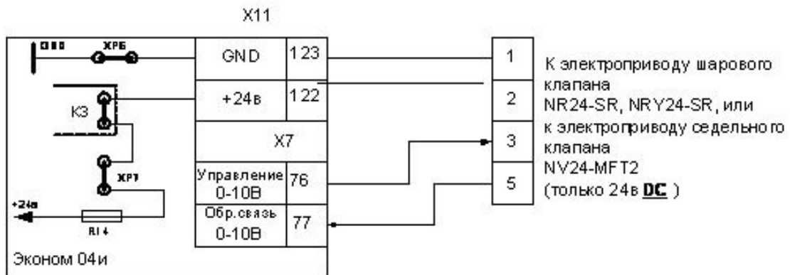
Рис. 6.13 – Схема подключения привода «Velimo» с аналоговым управлением 0-10В 2-го канала
