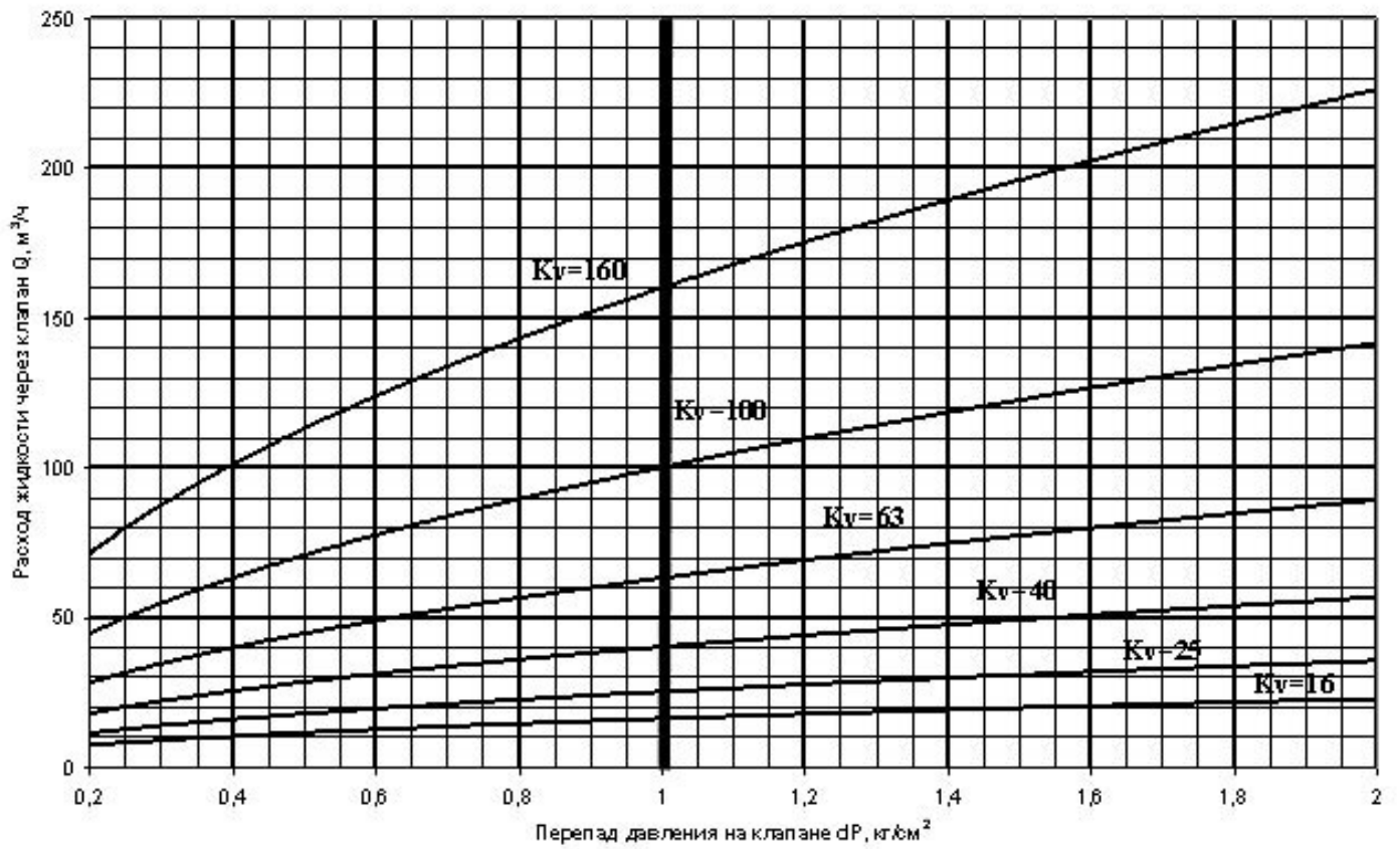
Рис. 3.3. Диаграмма подбора клапанов КС Ду50,80,100
