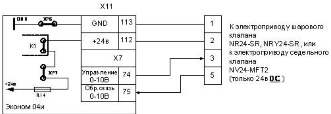
Рис. 6.12 – Схема подключения электропривода «Velimo» с аналоговым управлением 0-10В 1-го канала
