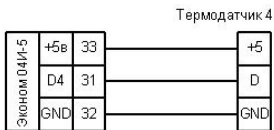
Рис. 9.4 – Схема подключения термодатчика 4
