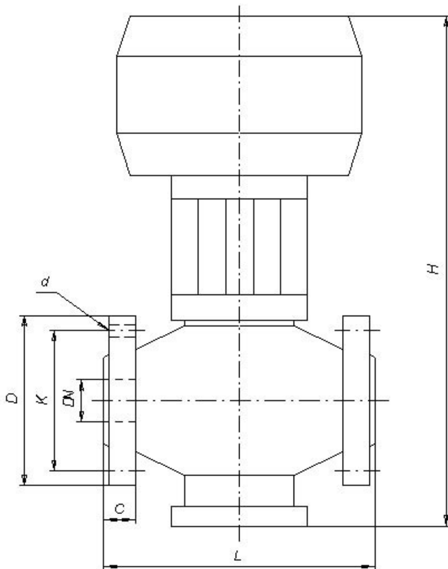
Рис. 3.4. Общий вид клапана КРС
