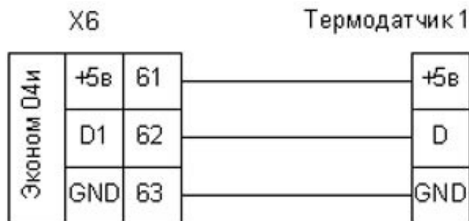
Рис. 6.1 – Схема подключения термодатчика 1
