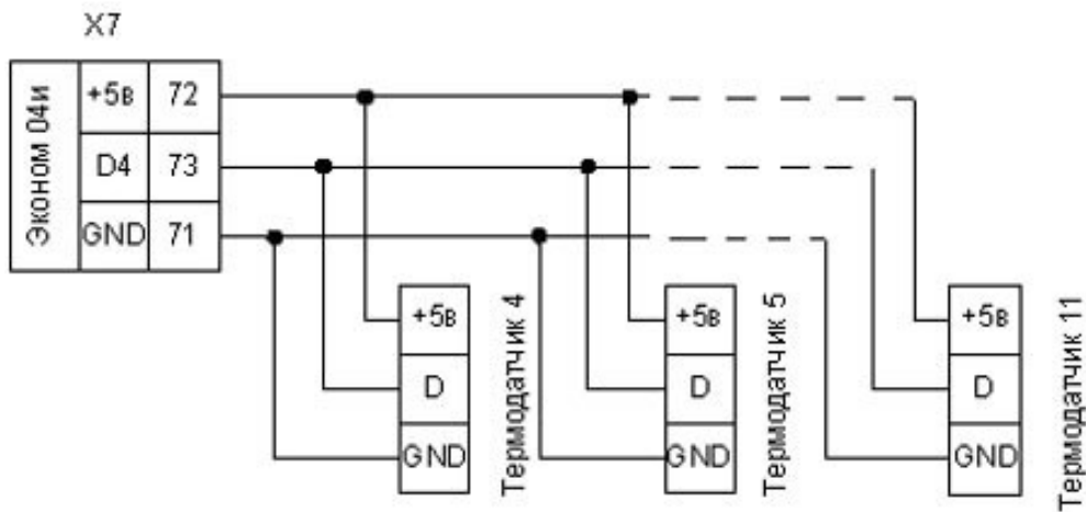
Рис. 6.5 – Схема подключения термодатчиков с шинной архитектурой
