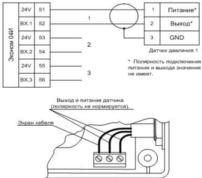
Рис.6.18 Схема подключения аналоговых датчиков 4-20 мА.
