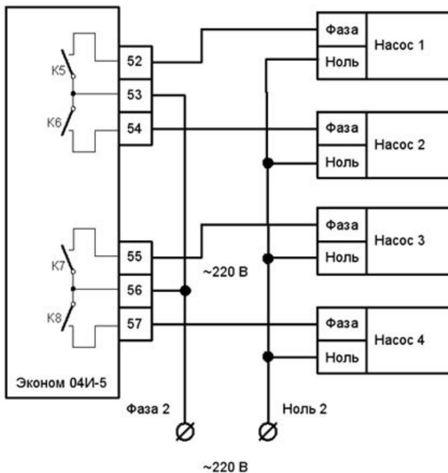
Рис. 9.17 – Схема подключения насосов
