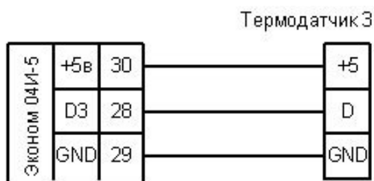
Рис. 9.3 – Схема подключения термодатчика 3
