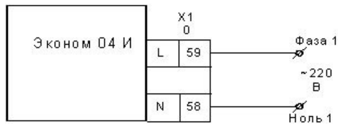
Рис. 6.16 – Схема подключения БУ к сети переменного тока ЦМУ 1,2
