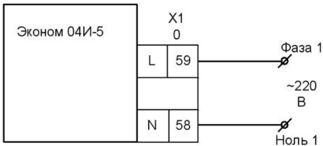
Рис. 9.16 – Схема подключения БУ к сети переменного тока
