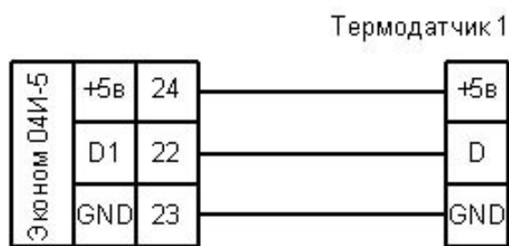
Рис. 9.1 – Схема подключения термодатчика 1
