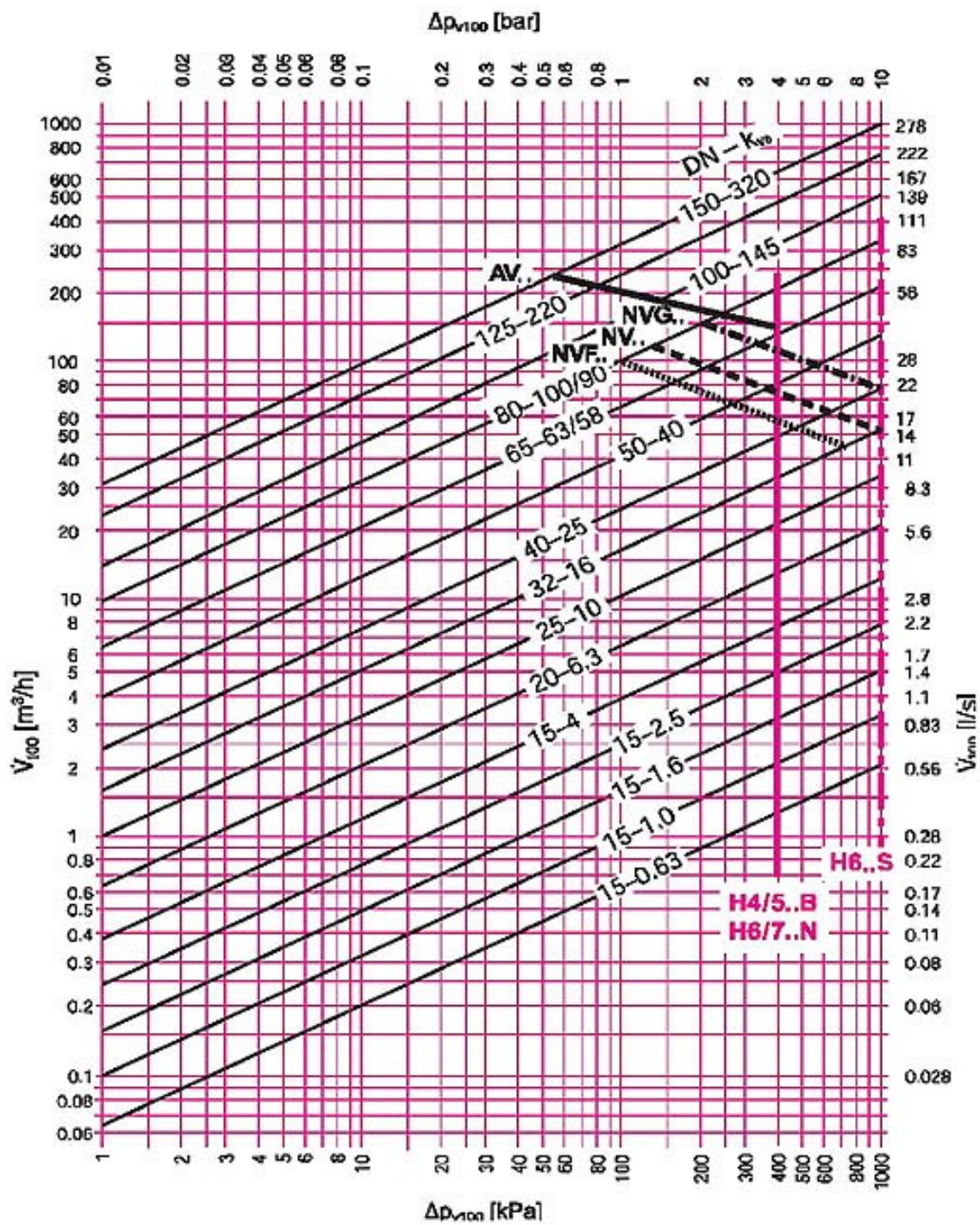
Рис. 3.5. Диаграмма подбора клапанов КРС, Н6..S
