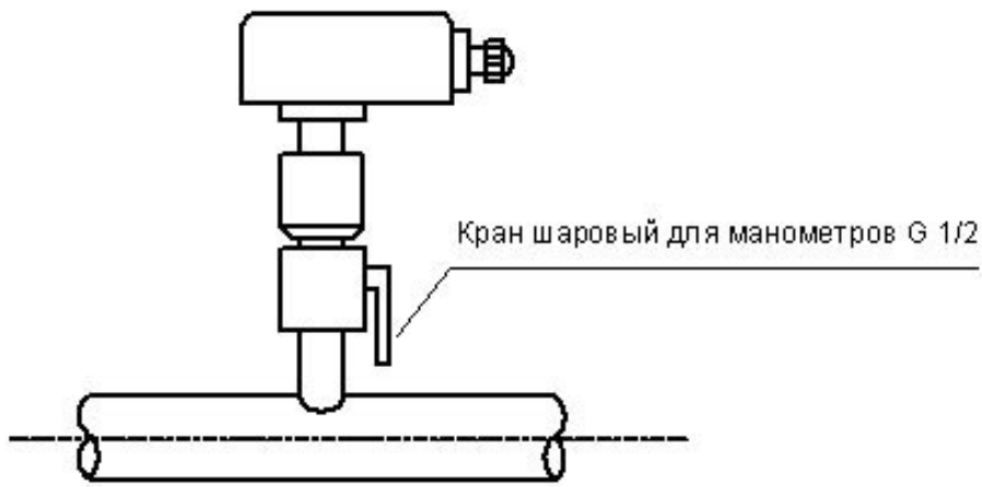
Рис.6.24 Установка датчика давления на трубопровод
