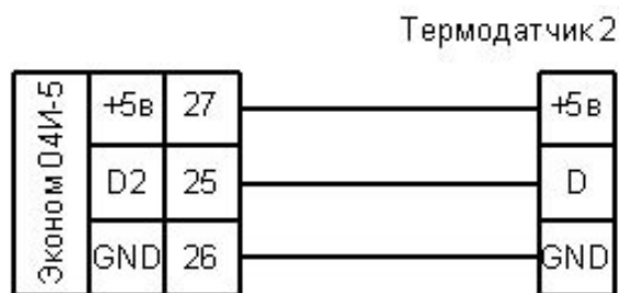
Рис. 9.2 – Схема подключения термодатчика 2
