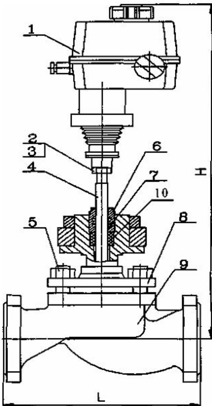
Рис. 3.1. Общий вид клапана КС
