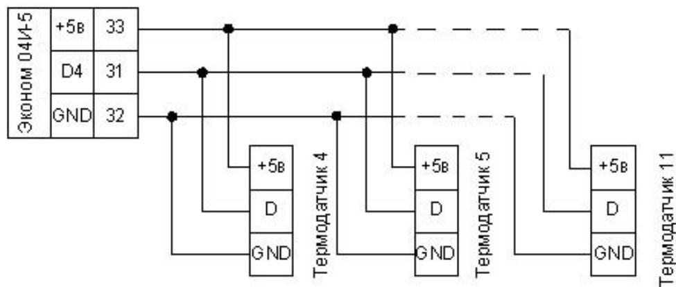
Рис. 9.5 – Схема подключения термодатчиков с шинной архитектурой
