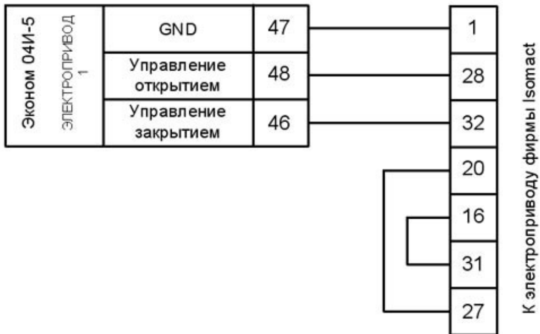
Рис. 9.8 – Схема подключения электропривода 220В «Isomact» с трехточечным управлением к 1-му каналу
