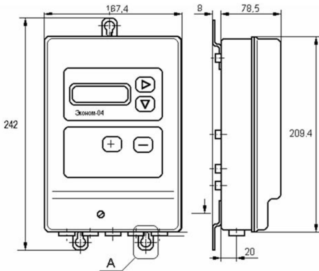
Разметка для крепления прибора
