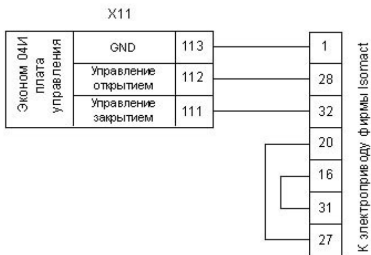
Рис. 6.8 – Схема подключения электропривода 220В «Isomact» с трехточечным управлением к 1-му каналу
