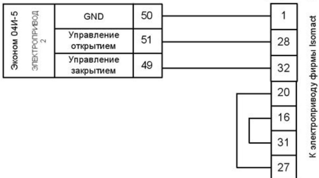
Рис. 9.9 – Схема подключения электропривода 220В «Isomact» с трехточечным управлением ко 2-му каналу
