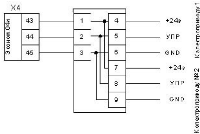
Рис. 6.15 – Схема клеммной коробки разветвления интерфейса МР для электроприводов «Belimo» с управлением МРТ (2)
