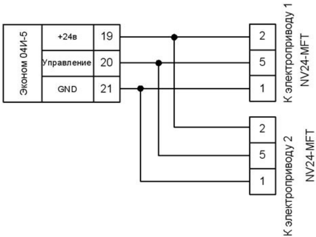
Рис. 9.14 – Схема подключения электроприводов «Belimo» с шинной архитектурой
