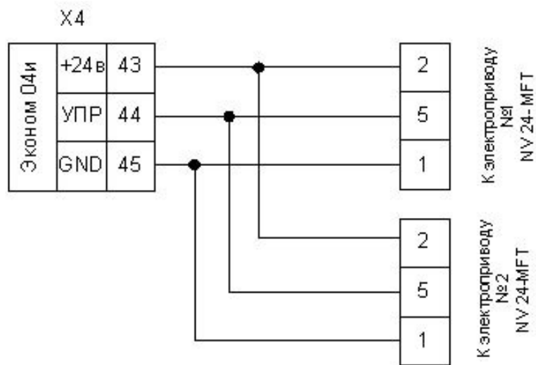
Рис. 6.14 – Схема подключения электроприводов «Belimo» с шинной архитектурой
