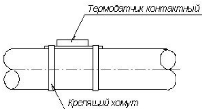
Рис. 6.20 – Схема установки термодатчика контактного на трубах
