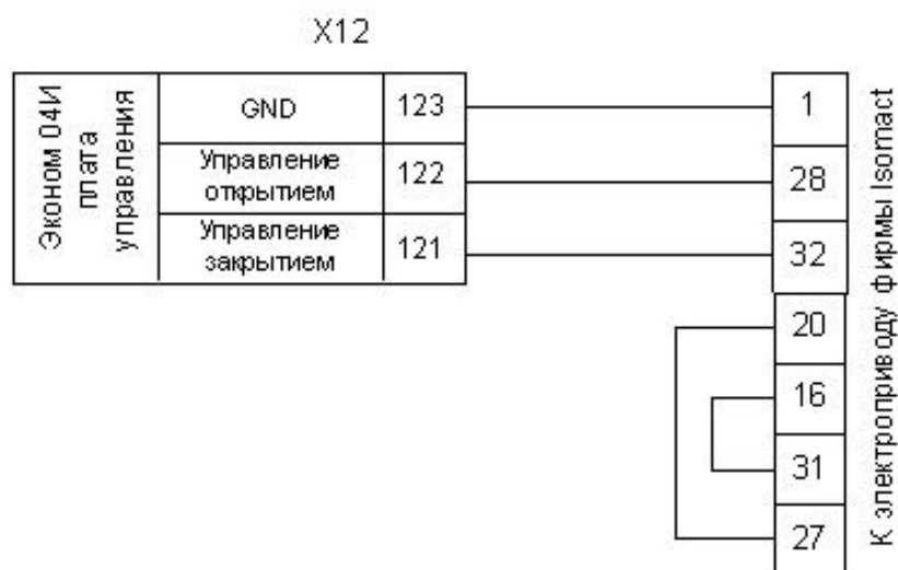
Рис. 6.9 – Схема подключения электропривода 220В «Isomact» с трехточечным управлением ко 2-му каналу
