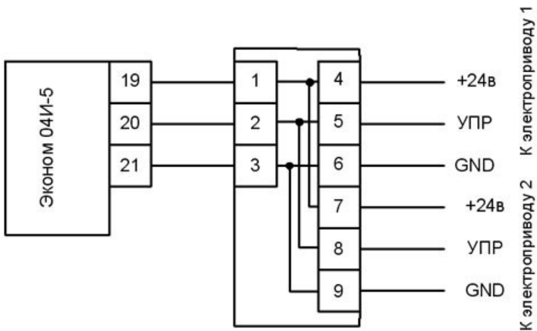
Рис. 9.15 – Схема клеммной коробки разветвления интерфейса МР для электроприводов «Belimo» с управлением МFT (2)
