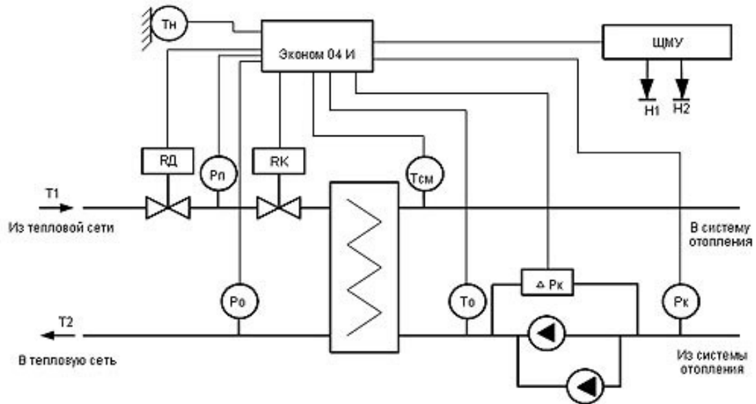
Рис. 1.2 Применение терморегулятора в независимой системе отопления с регулированием перепада давления.
