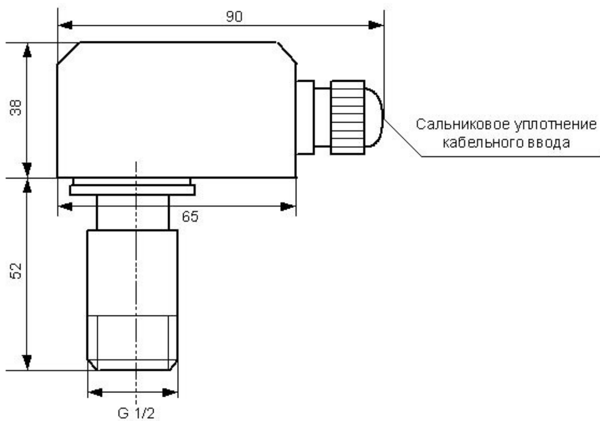
Рис.6.23 Внешний вид и габаритные размеры датчика давлен
