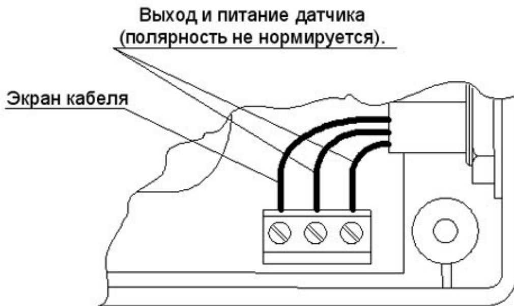
Рис.9.18 Схема подключения аналоговых датчиков 4-20 мА.
