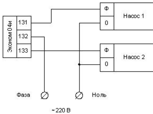
Рис. 6.17 – Схема подключения насосов
